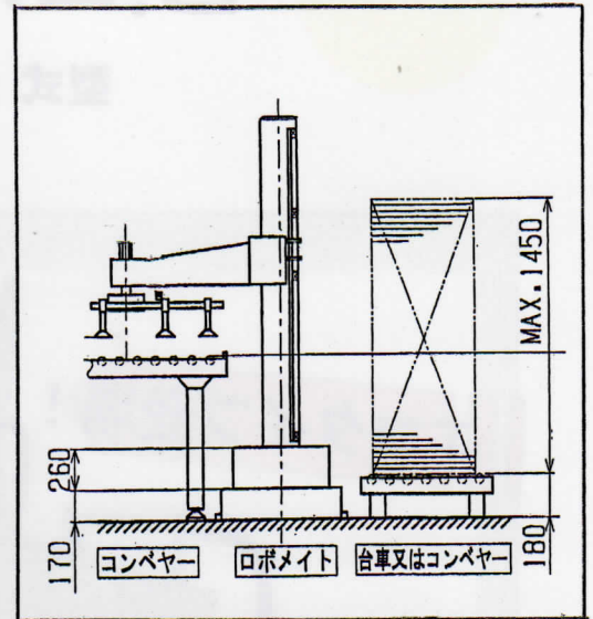
HRB側面図
